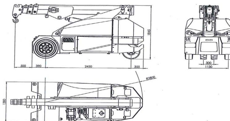
Fig. VII. Vues standard
